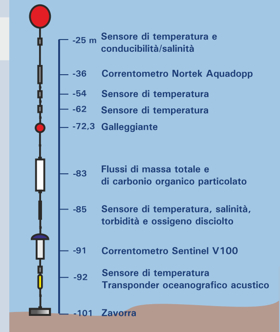
Schema del Mooring Dirigibile Italia
